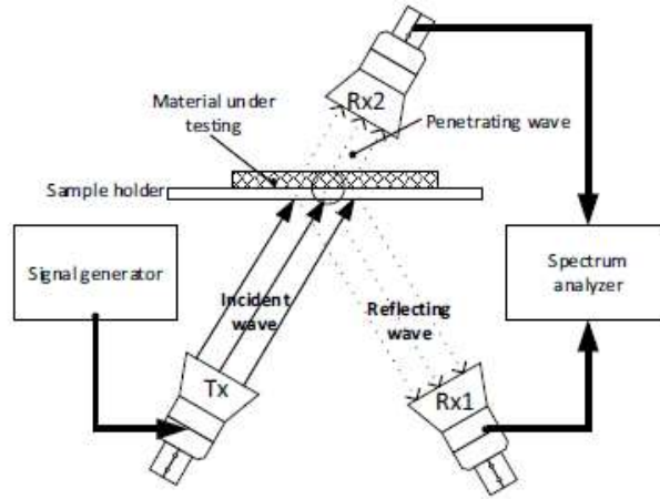
Şekil 2. Deney düzenegi
